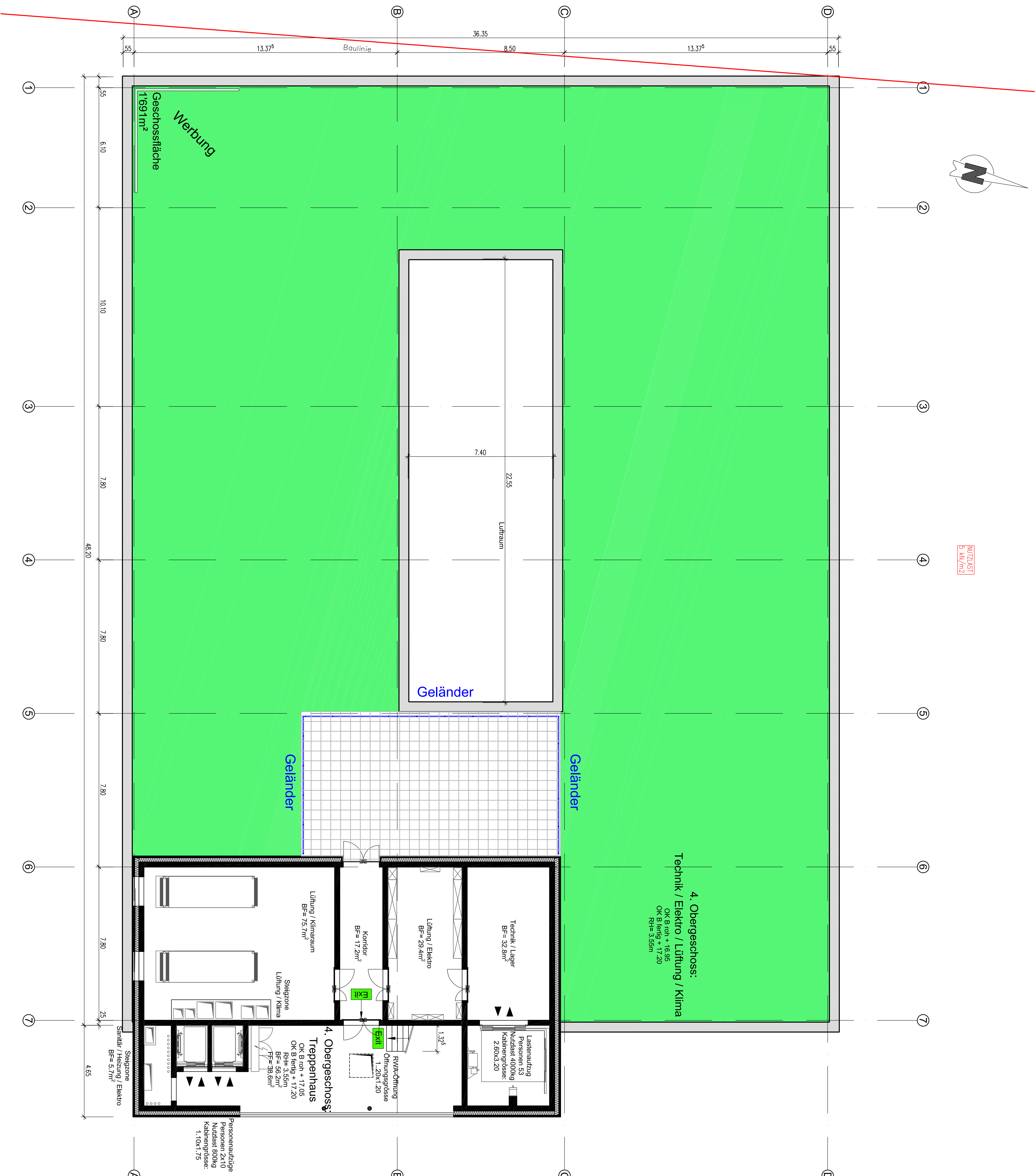
Grundriss 4. Obergeschoss Technik 1:100
